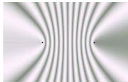
Рис.10 Сдвига фаз нет. Ориентация \vec{D} направлению перемещения ( \theta=0^\circ ) параллельная (движение осцилляторов слева направо). Скорость перемещения V=0,75c .
