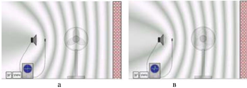
Рис.31 Появление потока воздуха между динамиком и стенкой (поток создаётся вентилятором) приводит к деформации интерференционной картины смещению контрольного узла в направлении стенки. Пакет стоячих волн сжимается.
