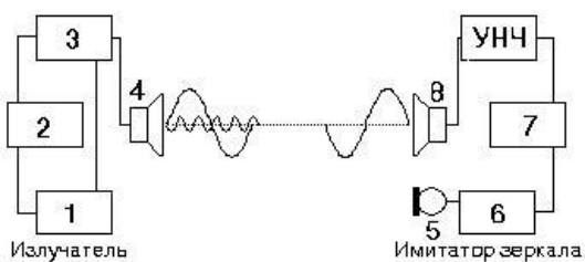
Рис.61 Блок-схема используемого в экспериментах прибора : 1 – звуковой генератор; 2 – умножитель частоты ( \times 4 ), служит для формирования пилот-сигнала; 3 – смеситель; 4,8 – динамики; 5 – микрофон для приёма пилот-сигнала; 6 – делитель частоты ( :4 ); 7 – восстановитель базового сигнала.
