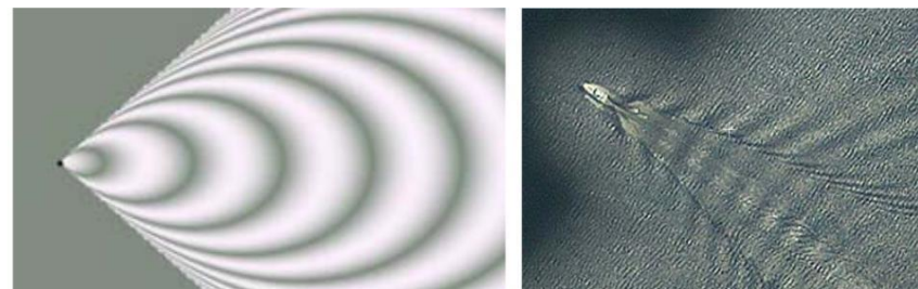
Рис.19 В сверхзвуковом конусе одиночного осциллятора возникает стоящее, относительно источника, поле волновой энергии. Скорость этого поля в точности равна скорости источника ( V=1,5c ), т.е. поле движется вместе с источником. На фото из космоса видна бегущая за катером волновая картина. Неверно!
