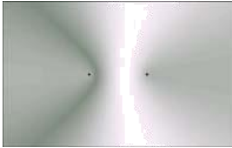
Рис.82 Сдвиг фаз между осцилляторами равен \Delta\phi = 45^\circ ( V=0 ), произошёл сдвиг стоячей волны вправо.
