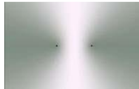
Рис.81 Так выглядит система осцилляторов ( V = 0 , \Delta\phi = 0^\circ ), у которой параметры сдвига фаз и скорости согласованы по правилу V = c \cdot \Delta\phi / \pi
