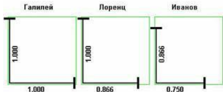
Рис.48 Длина плеч интерферометра зависит от выбора типа сокращений размеров. Расчёт приведён для V=0,5c .
