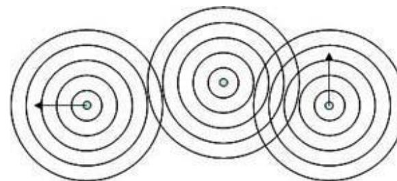
Рис.5 В геометрии без носителя нельзя обойтись одним рисунком, т.к. каждый осциллятор в зависимости от желания геометра вправе считаться началом отсчёта.
