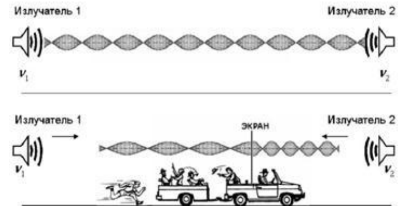
Рис.67 Излучатели когерентны ( v_1 = v_2 ). Стоячая волна движется вместе с экраном, её параметры изменились. Стоячая волна с изменёнными параметрами имеет место только для движущегося наблюдателя, поэтому мы назвали её «живой стоячей волной». Если наблюдатель изменит скорость, то изменятся и параметры стоячей волны.
