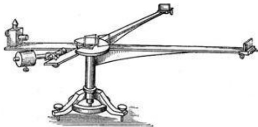
Рис.46 Общий вид первого интерферометра Майкельсона
