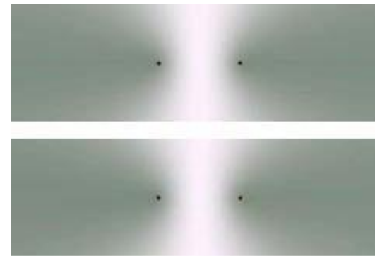
Рис.110 На верхней картинке сдвиг фаз отсутствует ( \Delta\phi = 0^\circ ), а на нижней – \Delta\phi = 1^\circ , что соответствует скорости системы V = 1666,6 \text{ км / с} . Для глаза картинка различима с трудом.
