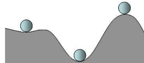
Рис.86 Зоны устойчивого (потенциальные ямы) и неустойчивого равновесия.
