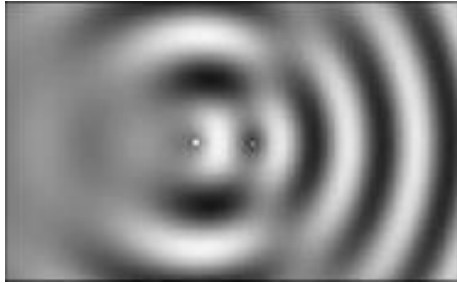
Рис.39 Произошло нарушение внутреннего равновесия. Появилось излучение вонне ( V > 0 , \square\phi = 0 , l=1 ).
