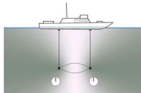
Рис.104 Аналог эксперимента Бьеркнеса.
