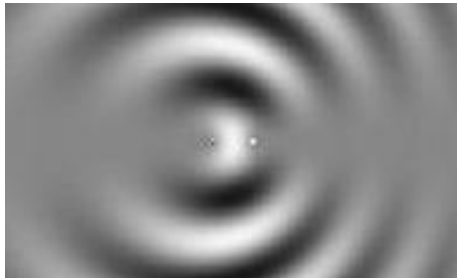
Рис.40 Благодаря произведённым изменениям ( V > 0 , \square\phi = \pi \cdot V / c , l = 1 \cdot (1 - \beta^2) ) внутреннее равновесие системы восстановилось.
