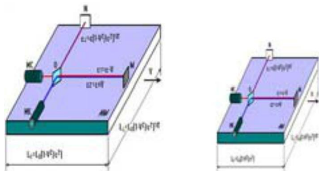
Рис.55 Изменение размеров интерферометра по Лоренцу (слева) и в соответствии со сжатием стоячих волн (справа).
